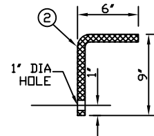
SECTION D-D
